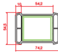
54X80 Kutu 54x80 Box
