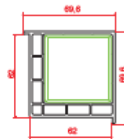
62X62 Kutu 62x62 Box
