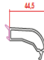
4mm Cam Çıtası 4mm Glass Bead
