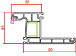
Süper Pervazlı Kasa Super Architrave Frame
