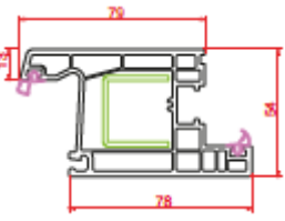
Kapı Kanat Door Sash
