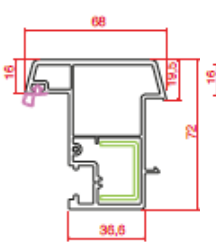
Hareketli Ortakayıt Narrow Mullion
