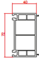
72 mm 4 cm Yükseltme 72 mm 4 cm Extension
