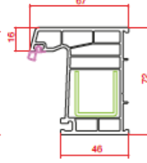
Süper Kasa Super Frame
