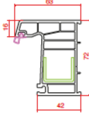
Kasa Frame
